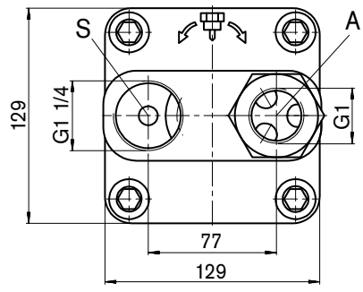
Ansicht X
