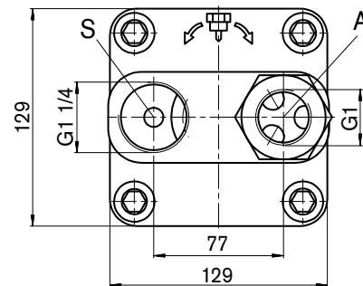
Ansicht X
